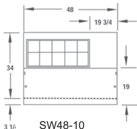
SW48-10
