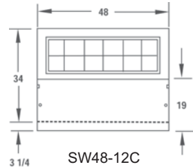
SW48-12C
