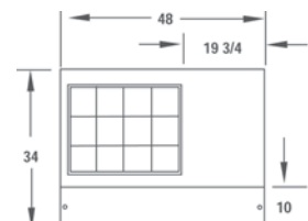
SW48-12M
